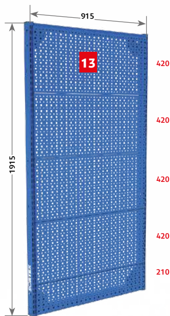
Система хранения SORTEX 1915-S №1-1
