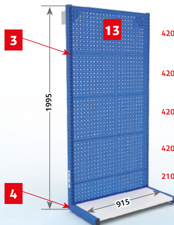
Система хранения SORTEX 1915-1 №1-1
