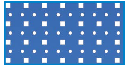
Универсальная перфорация стенок (квадрат 10 мм, шаг 38х38 мм; круг 7 мм, шаг 25х38 мм)
