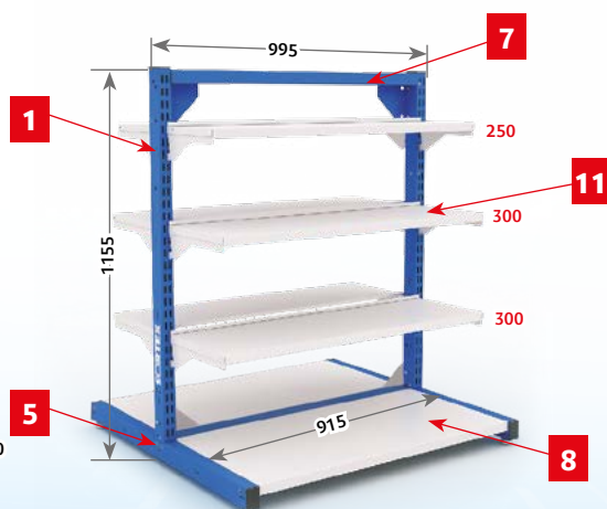
Система хранения SORTEX 1075-2 №1-1
