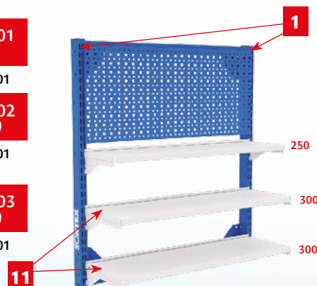
Система хранения SORTEX 1075-S №1-2
