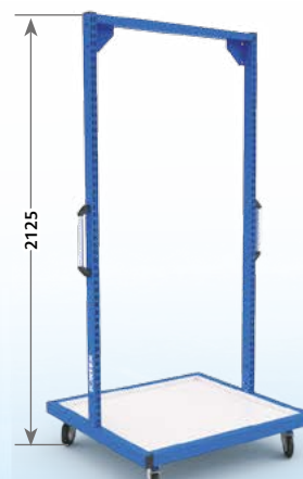
Система хранения SORTEX 1915-M Base
