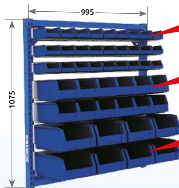
Система хранения SORTEX 1075-S №1-1
