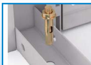
Анкерное крепление к полу
