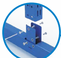
Узел крепления стойки к опоре
